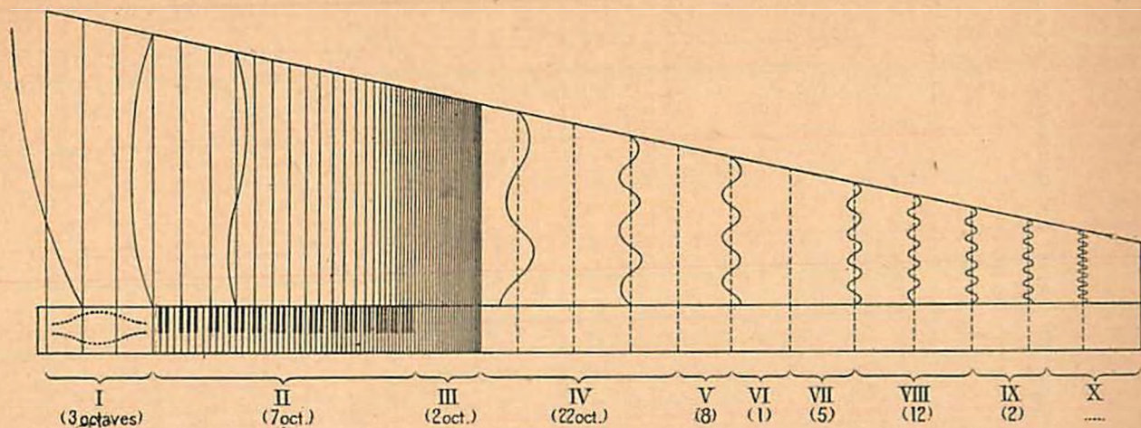
Fig. 17. — Échelle des fréquences de vibration ou clavier des ondes de l'univers : I, fréquences industrielles (3 octaves) ; II, fréquences musicales (clavier du piano 7 octaves) ; III, ondes ultra-sonores (2 octaves) ; IV, ondes radioélectriques (22 octaves) ; V, ondes infrarouges (8 octaves) ; VI, ondes lumineuses (1 octave) ; VII, ondes ultraviolettes (5 octaves) ; VIII, rayons X (12 octaves) ; IX, radioactivité (6 octaves, dont \frac{1}{4} communes avec les rayons X) ; X, rayons pénétrants.
