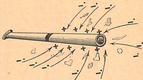
Fig. 5. — En frottant le fume-cigarette d'ambre, on lui enlève une certaine quantité d'universon, c'est-à-dire d'électrons ou de grains d'électricité négative. Autrement dit, on charge positivement le fume-cigarette. Les électrons négatifs accourent du dehors pour neutraliser cette électrisation et entraînent dans leur course les objets légers, papiers et fétus, qui se précipitent sur le fume-cigarette.
